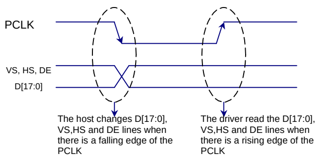
Fig. 9.9.1 PCLK cycle
