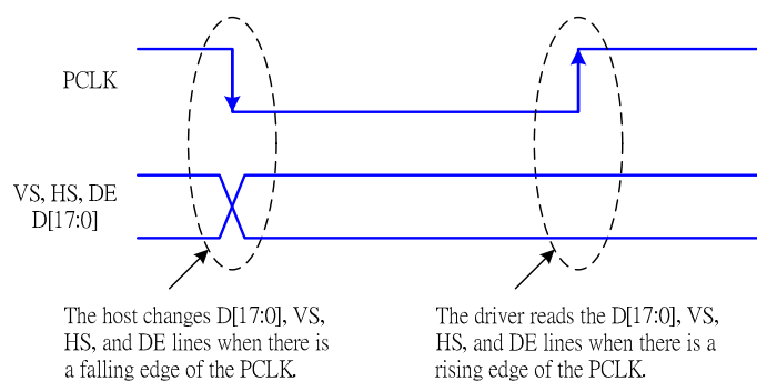
Fig. 9.9.1 PCLK cycle
