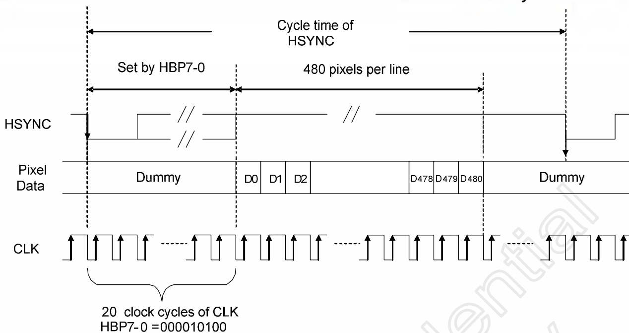
Fig 21. Horizontal Data
