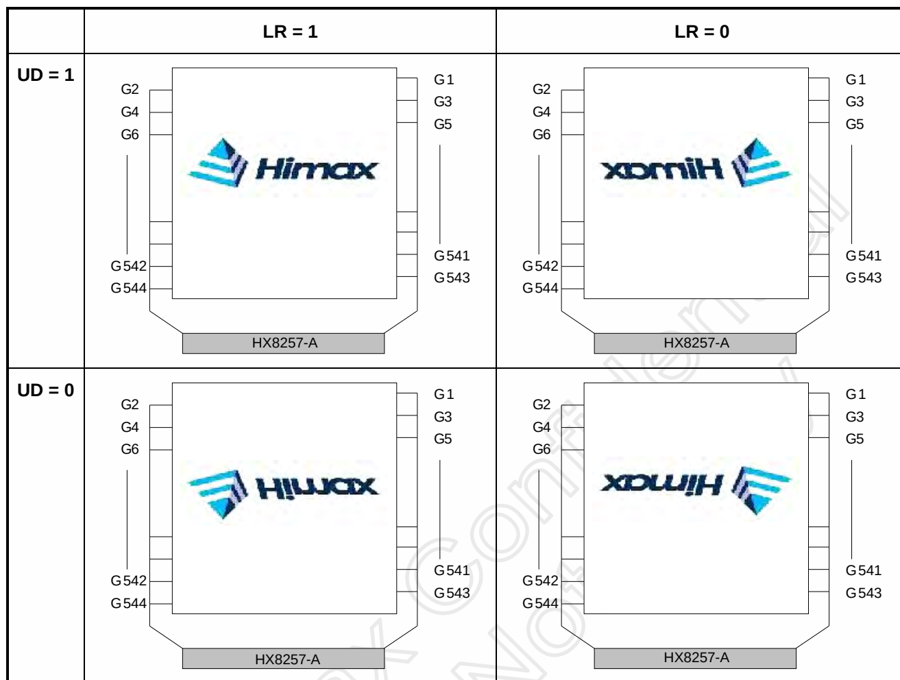
Fig 15. LR/UD Function
