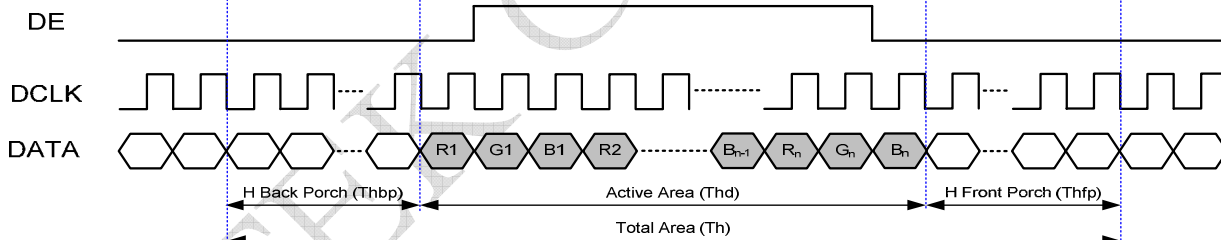
Serial RGB input timign table
