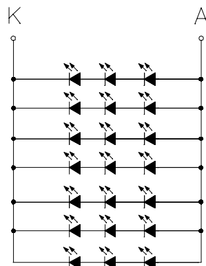
LED 电路图
